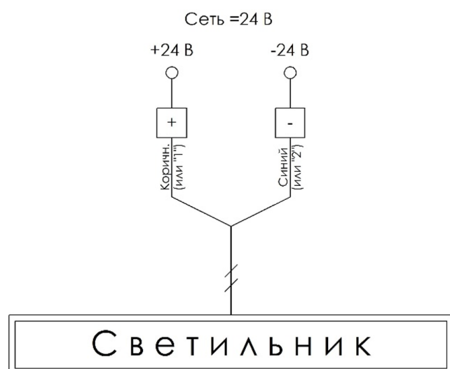
Схема подключения светильника с напряжением питания DC 24 В без функции управления
