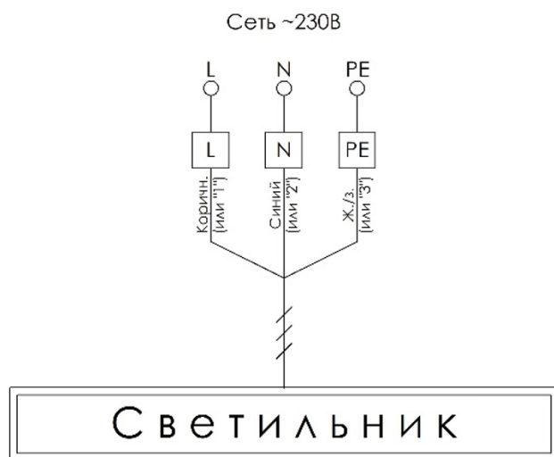
Схема подключения светильника с напряжением питания AC 230 В, (50±1) Гц, без функции управления
