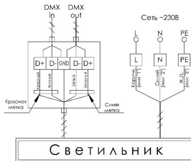
Схема подключения светильника с напряжением питания AC 230 В, (50±1) Гц с функцией управления DMX, RDM
