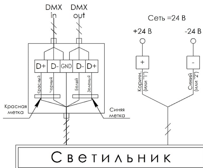
Схема подключения светильника с напряжением питания DC 24 В с функцией управления DMX, RDM
